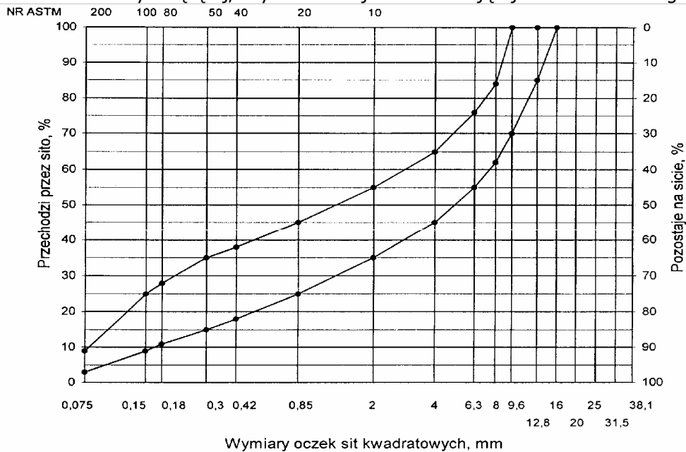
Rys. 9. Krzywe graniczne uziarnienia mieszanki mineralnej BA od 0 do 16 mm do warstwy wiążącej, wyrównawczej i wzmacniającej nawierzchni drogi o
